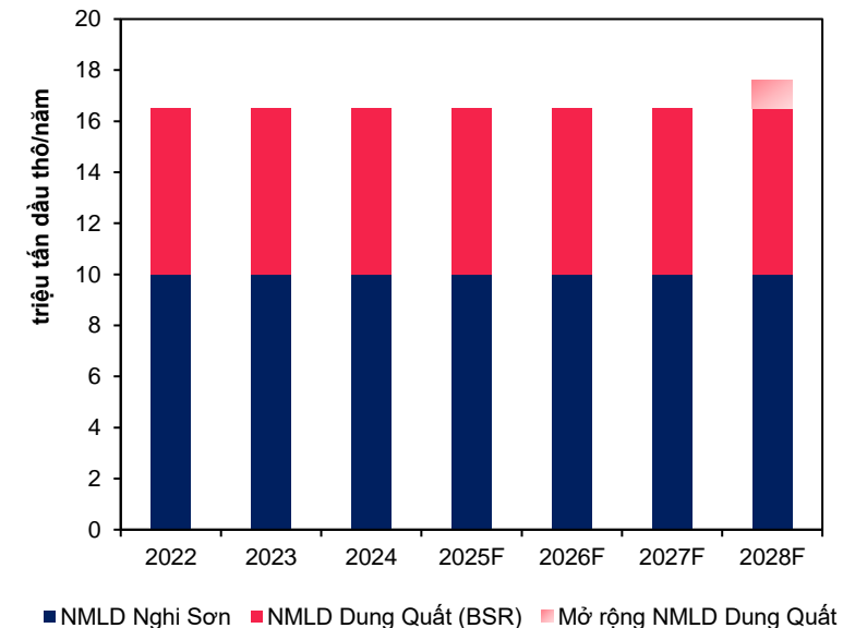
Công suất lọc dầu của VN dự kiến đi ngang đến 2028
